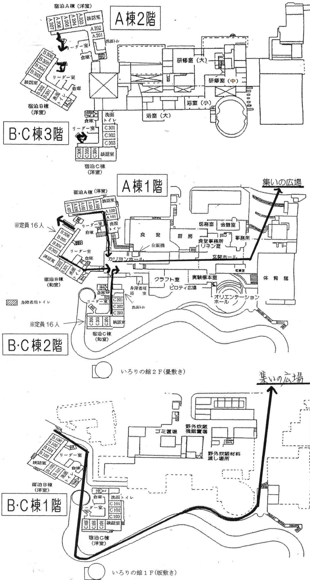
避難経路図 1
